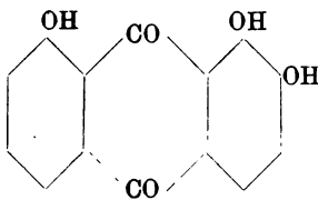
Oxychryszazin 1 : 2 : 8
